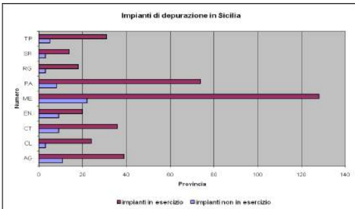
Grafico 2 – IMPIANTI DI TRATTAMENTO DELLE ACQUE REFLUE URBANE IN SICILIA
