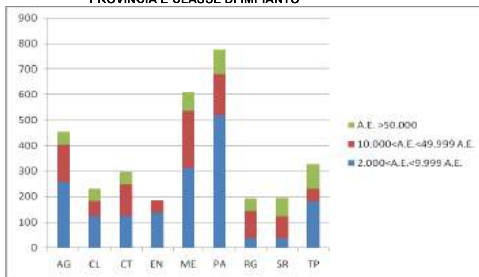
Grafico 4 - CONTROLLI DEGLI SCARICHI OBBLIGATORI DEL 2018 PER PROVINCIA E CLASSE DI IMPIANTO*
